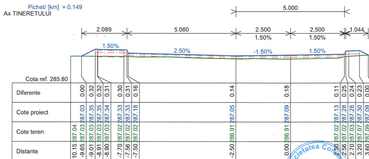
PROFILE TRANSVERSALE CARACTERISTICE Ax TINERETULUI Scara oriz. 1:100 vert. 1:100
